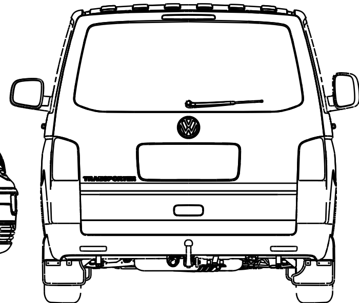
T5 Modelljahr / model year 2004-2009 Kombi mit Schiebetür rechts / with sliding door right kurzer Radstand / short wheelbase normale Dachhöhe / normal roof 1:25
