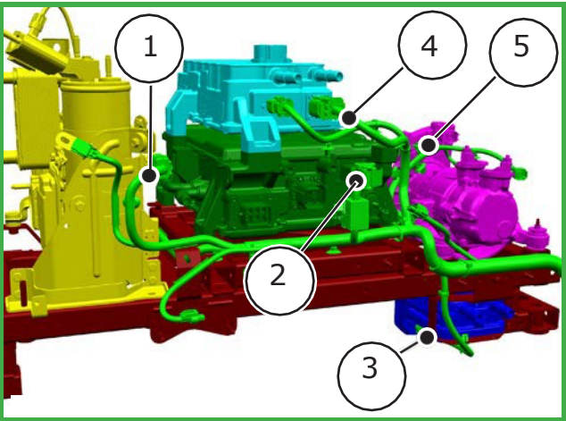
Connettore a basso voltaggio: parte anteriore del blocco ad alto voltaggio – veicolo elettrico
