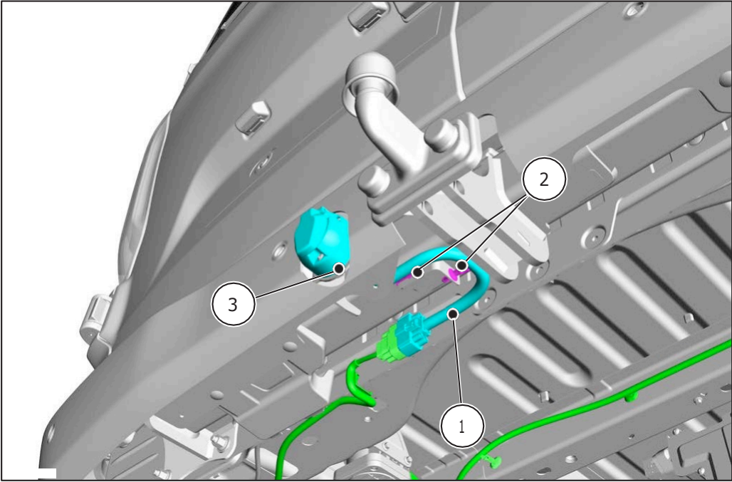
Kit di cablaggio, impianto elettrico per gancio a testa sferica (n. PR 1M5)
