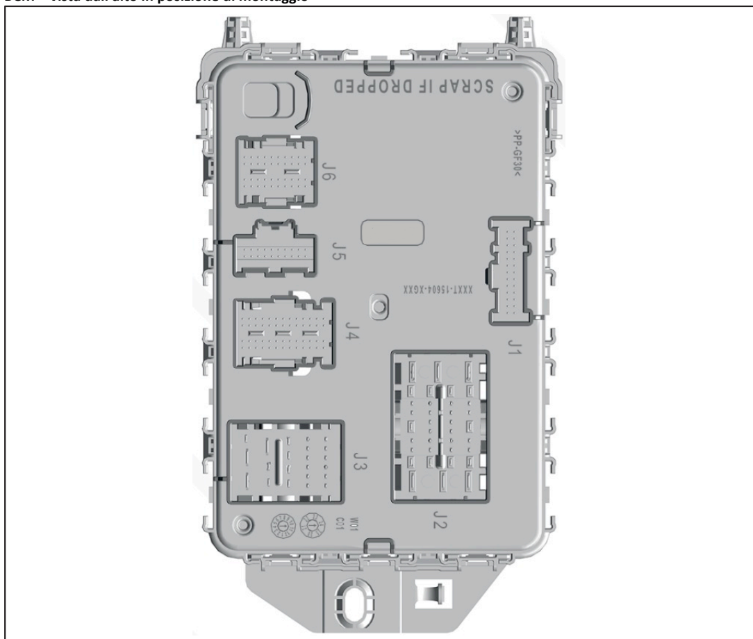
BCM – vista dall'alto in posizione di montaggio
