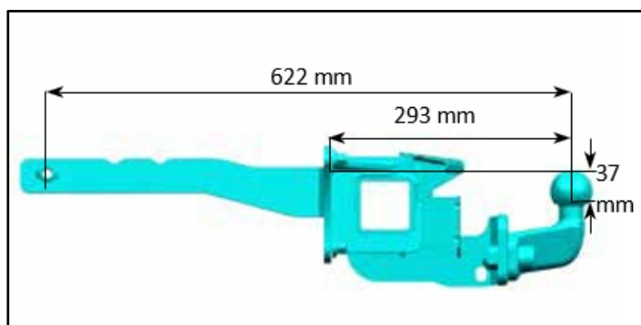
Fig. 2: gancio a testa sferica avvitato in modo fisso
