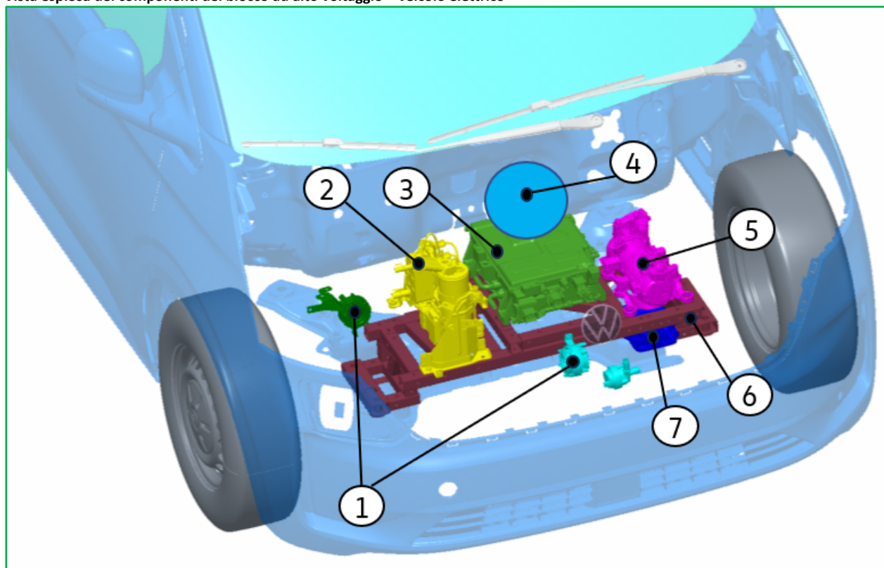
Vista esplosa dei componenti del blocco ad alto voltaggio – veicolo elettrico
