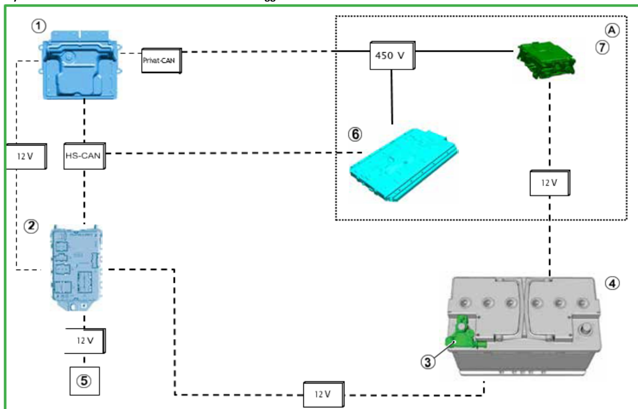
Layout del sistema di carica della batteria a basso voltaggio – veicolo elettrico
