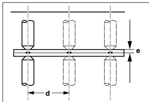
Verhältnis Blechdicke / Abstand der Schweißpunkte
