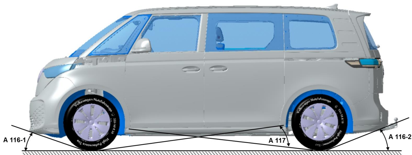
Abb. 1: Fahrzeugmaße exemplarisch ID Buzz People (gemäß DIN70020, T1)
