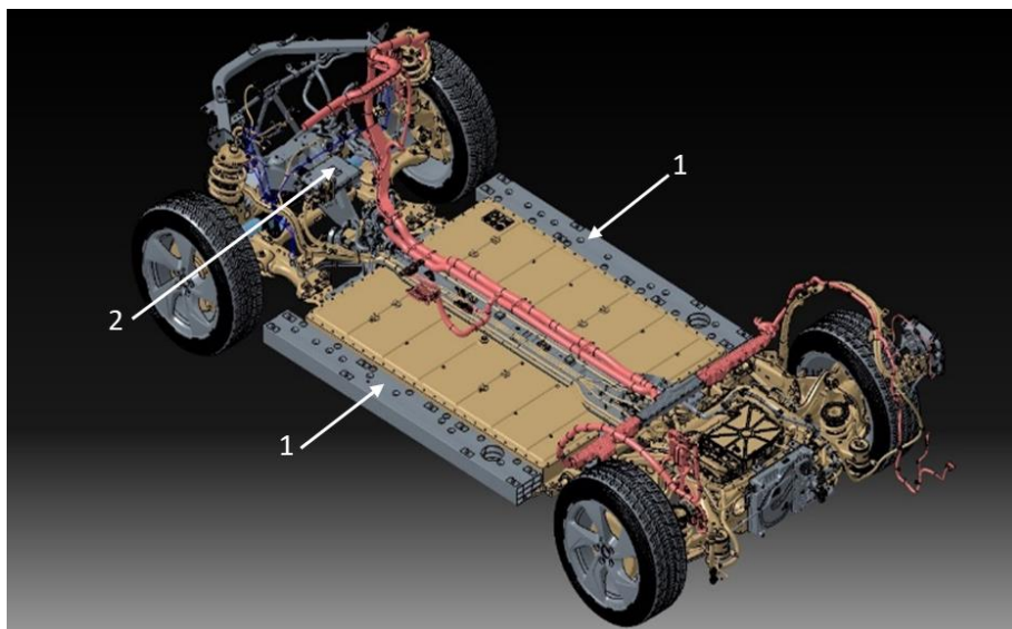
Abb. 2 Fahrzeugstruktur mit Batterie (82 kWh) und Zuleitung sowie Antriebseinheit für 150 kW Heckantrieb
