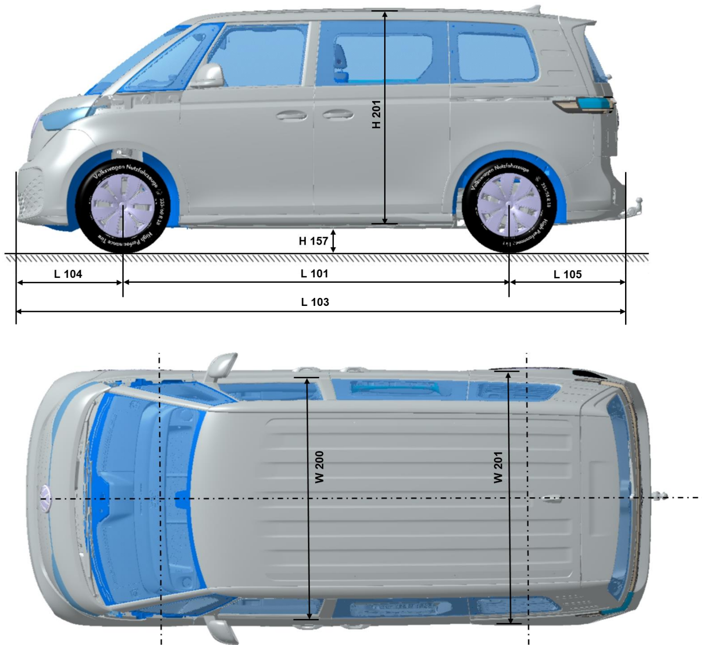
Abb. 1: Fahrzeugmaße exemplarisch ID Buzz People (gemäß DIN70020, T1). Die Maße finden Sie in unten stehender Tabelle Basisdaten.
