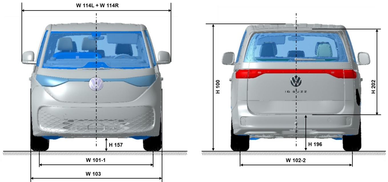
Abb. 2: Fahrzeugmaße exemplarisch ID Buzz People (gemäß DIN70020, T1) Die Maße finden Sie in unten stehender Tabelle Basisdaten.
