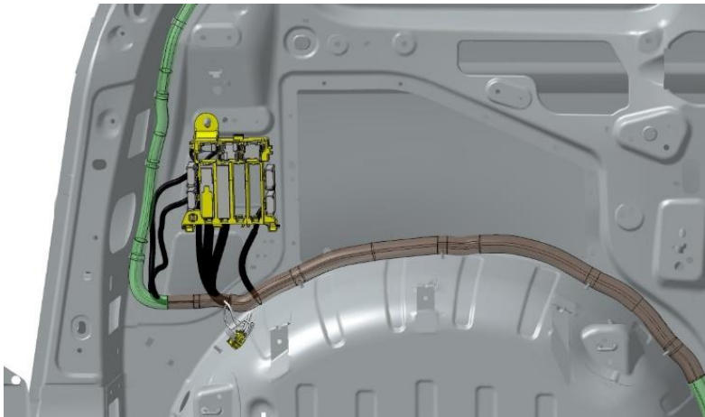
Abb.1: Sicherungsträger an der Seitenwand hinten links und Massepunkt auf dem Radkasten links.
